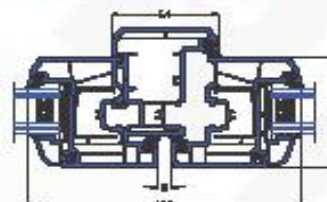
SECCIÓN CENTRAL
